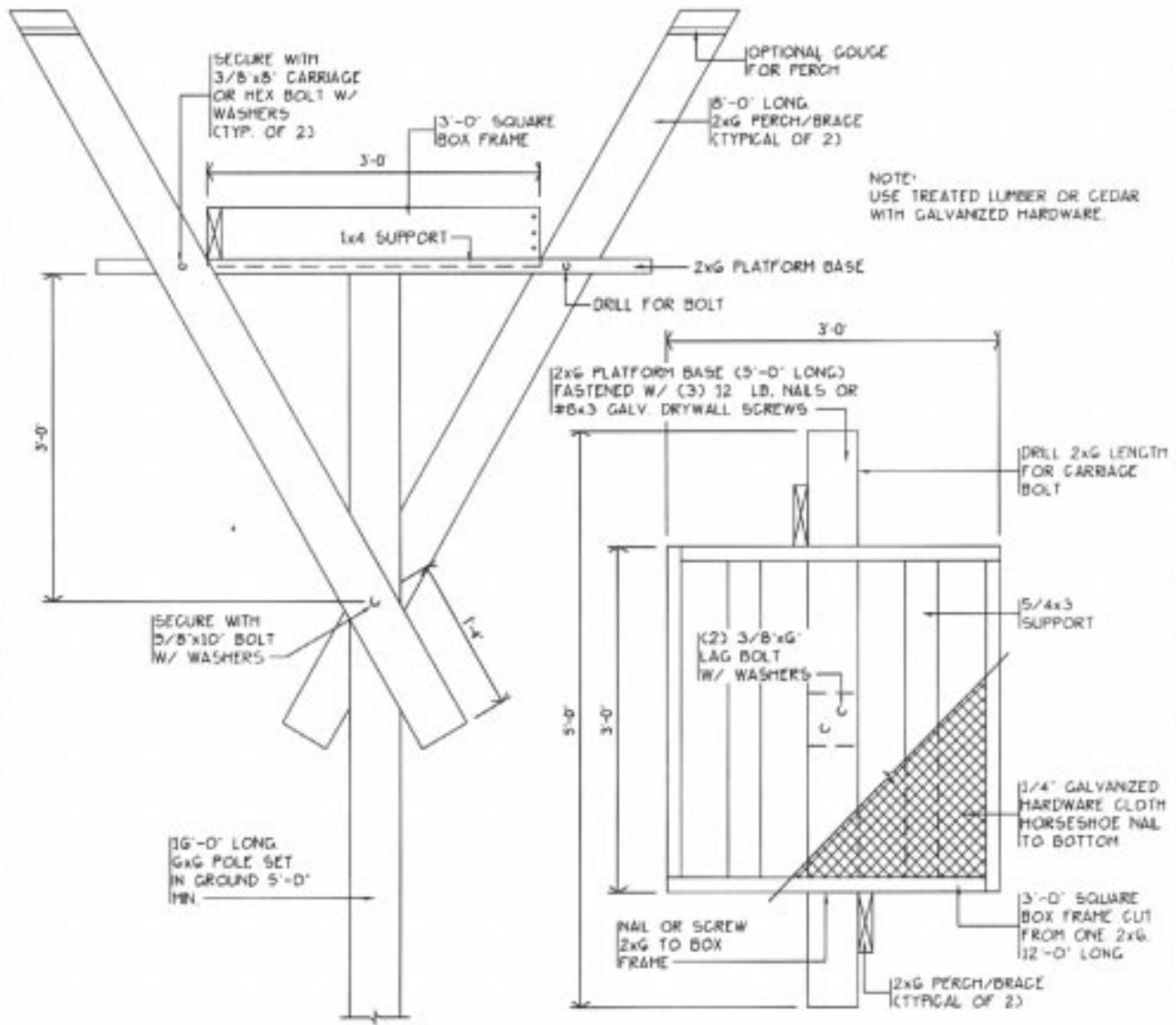
ELEVATION
